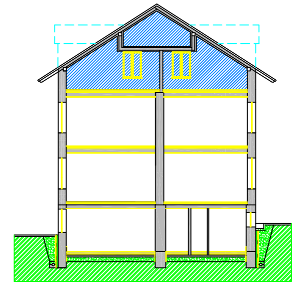
PREREZ A-A M 1:230
