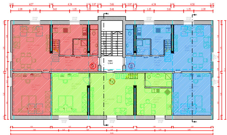
TLORIS MANSARDE M 1:230
