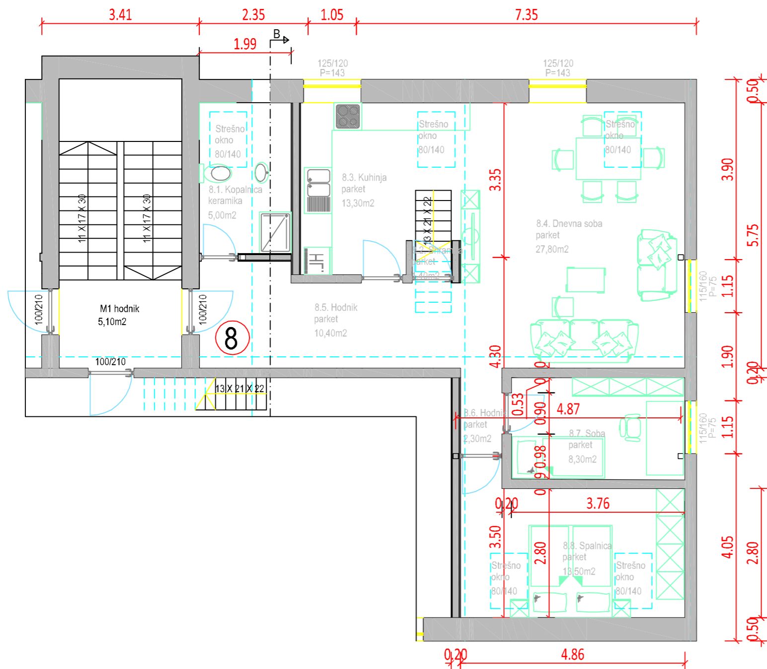
TLORIS MANSARDE M 1:80
