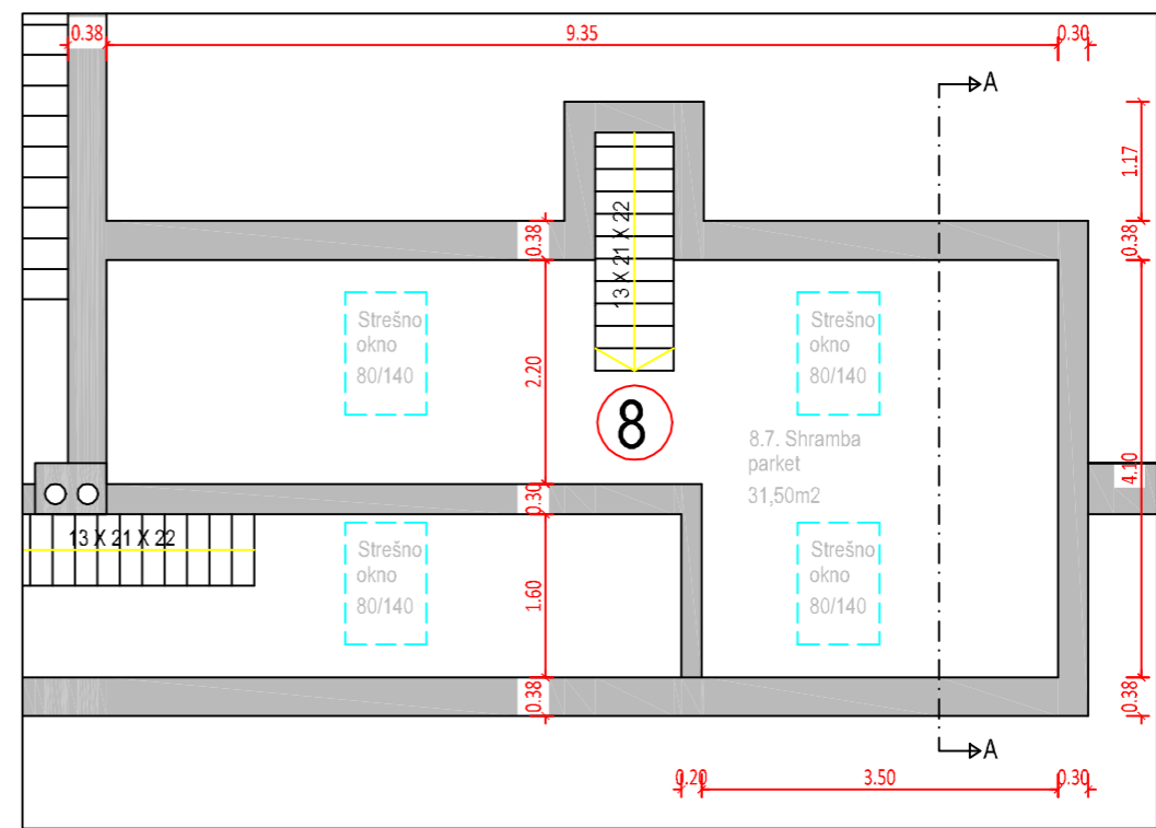
TLORIS GALERIJE M 1:80
