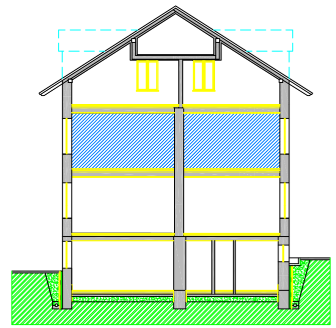
PREREZ A-A M 1:200
