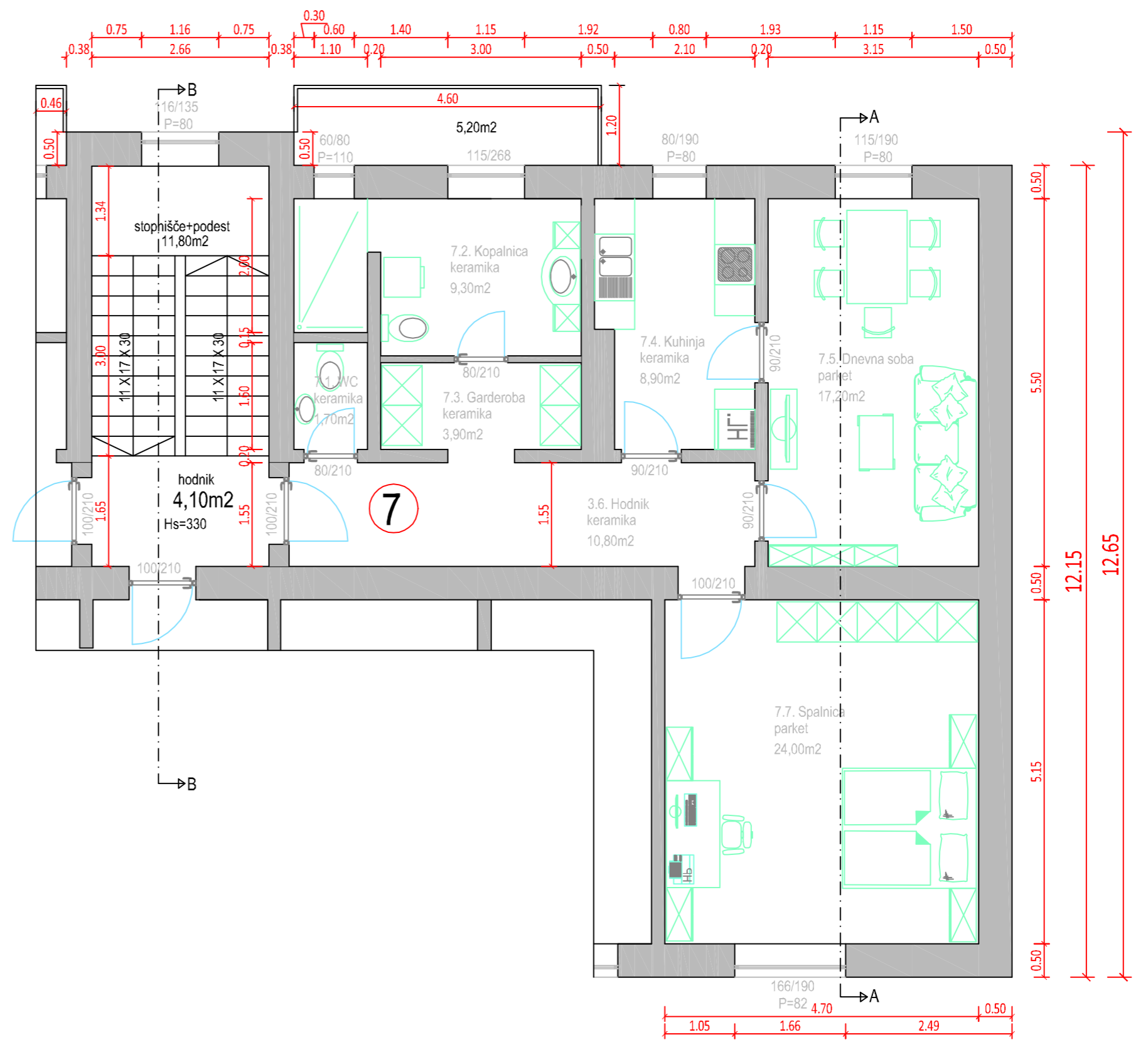
TLORIS NADSTROPJA M 1:70
