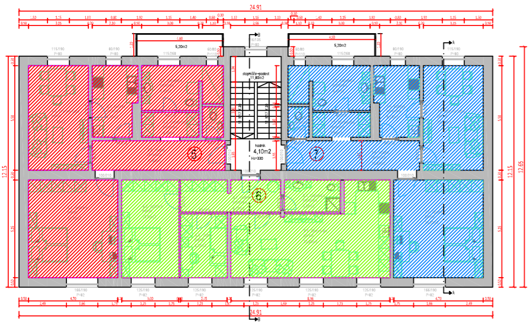
TLORIS NADSTROPJA M 1:200
