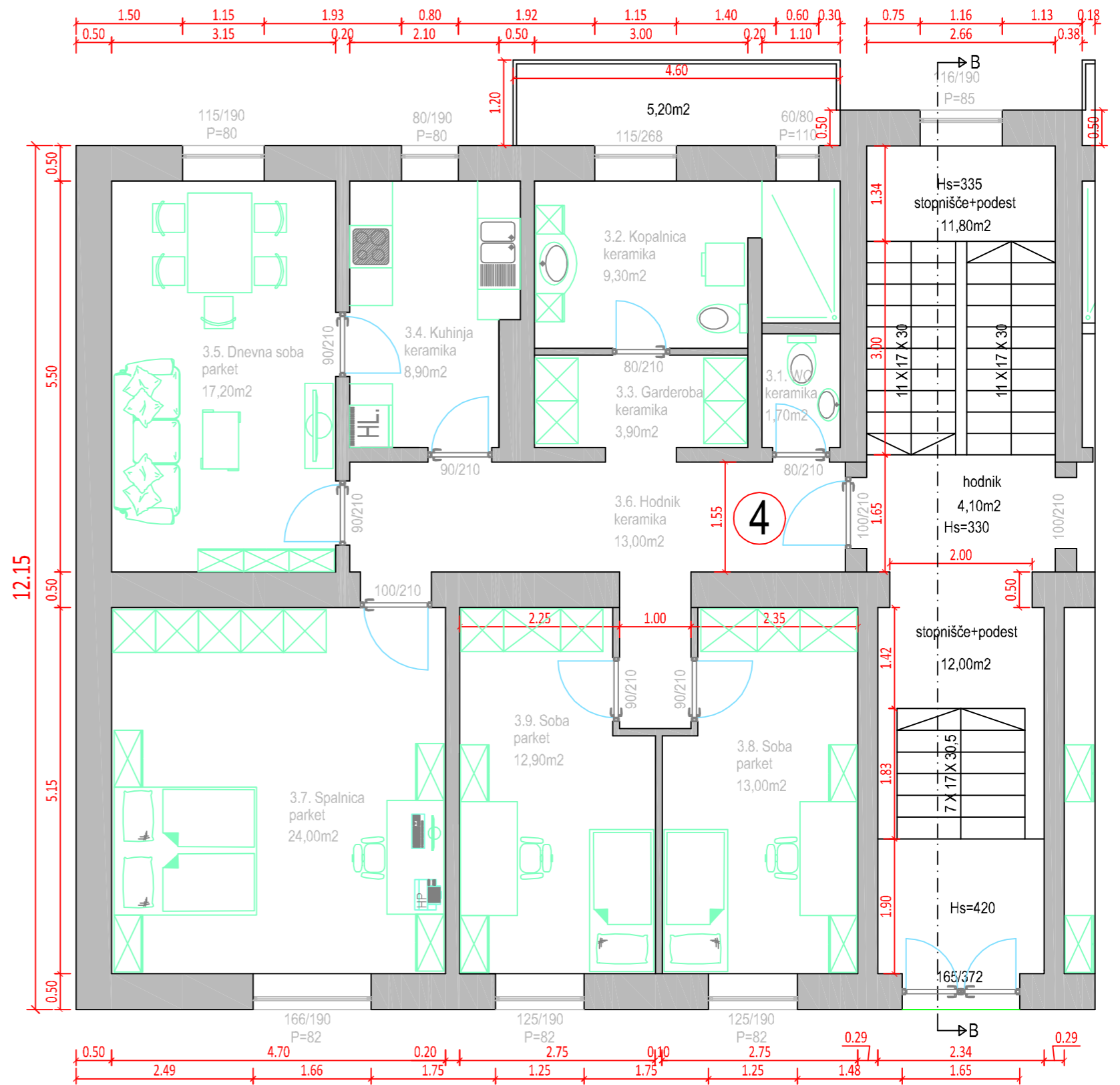
TLORIS PRITLIČJA M 1:70
