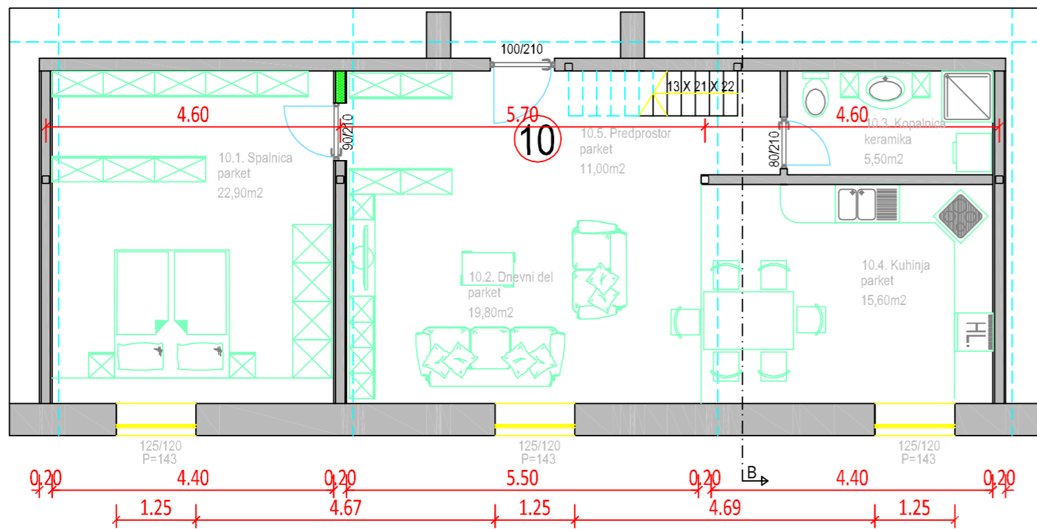
TLORIS MANSARDE M 1:80
