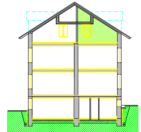
PREREZ A-A M 1:230
